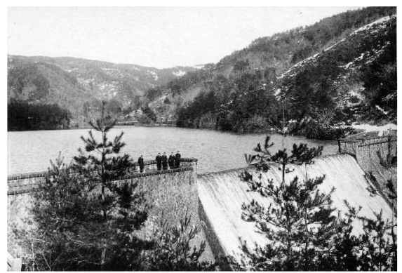
■ コンクリートダムとして復旧（大正11年）
